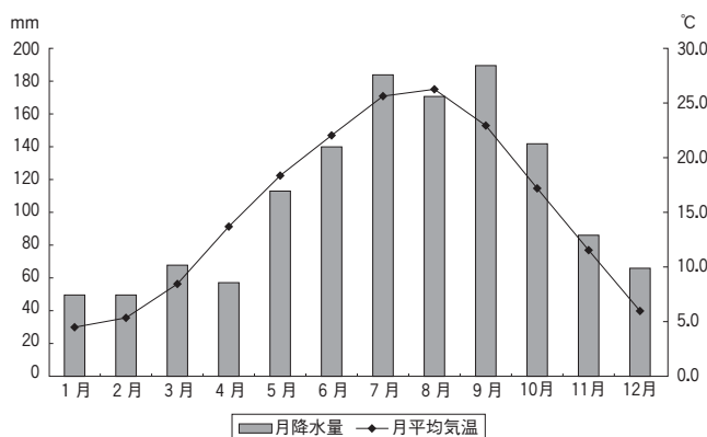
「阿波町・吉野町」の気象（2000～2009年の月別平均値） 穴吹観測所
