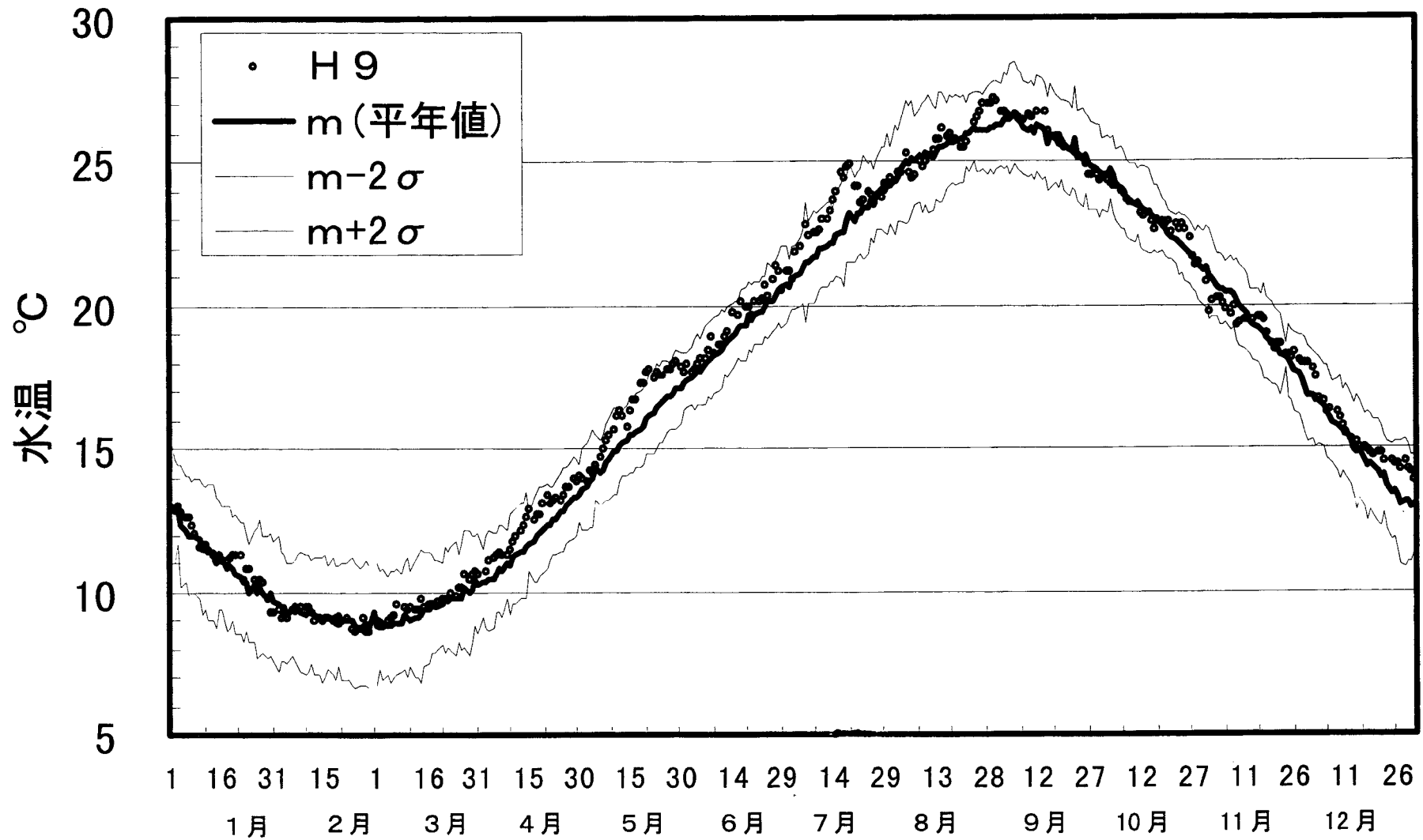
平成 9 年の鳴門分場汲み上げ海水温の日変化と平年値
