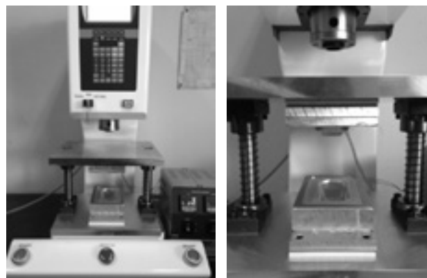
システム全体 加熱ヒーター・絞り金型
