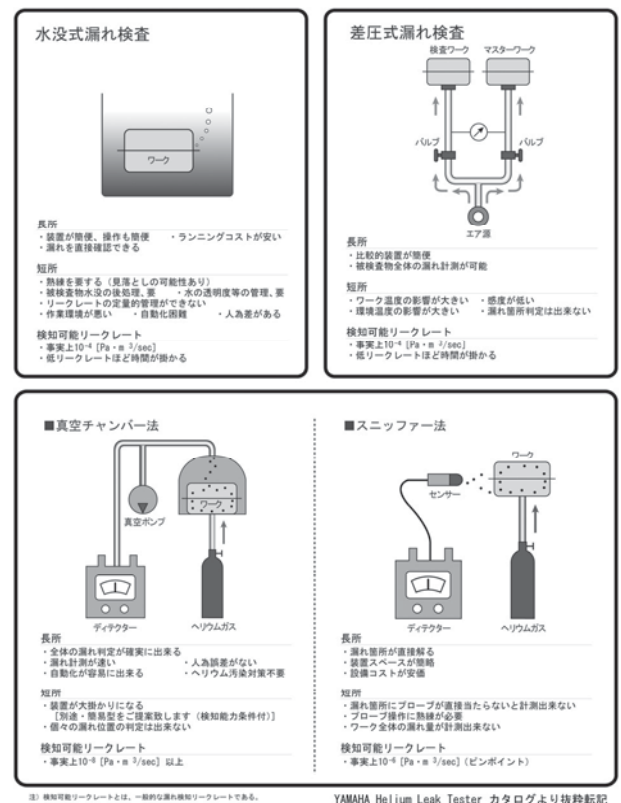
図1 リークテスト方式の特徴
