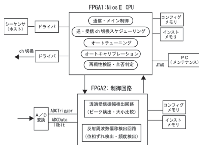
図6 信号処理回路基板とFPGAのブロック図
