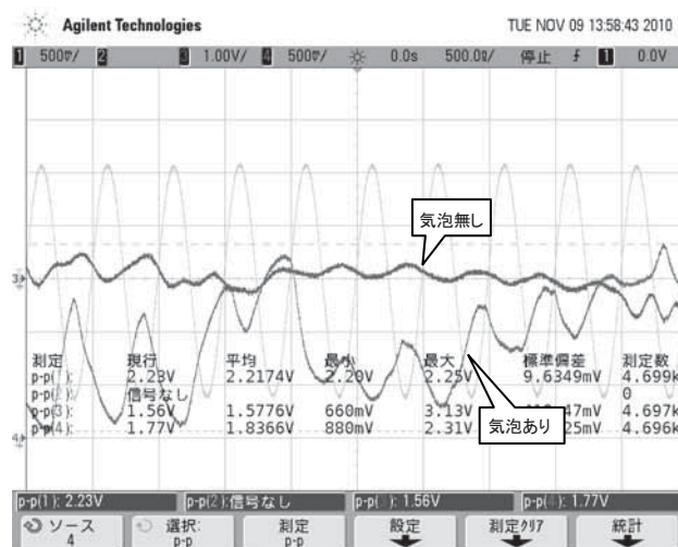
図9 気泡の有無による反射波の変化
