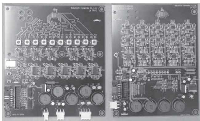
図5 製作した送(左)・受信(右)回路基板
