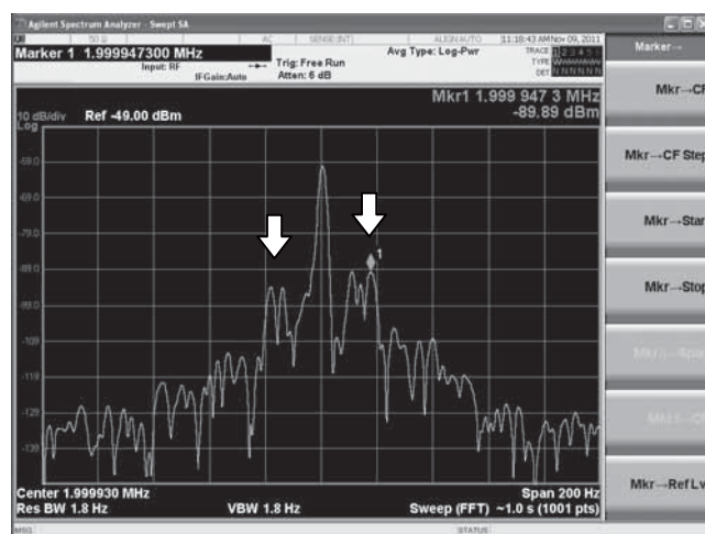
図10 \phi 0.1 \sim 0.2 \text{ mm} の気泡によるパワースペクトル
