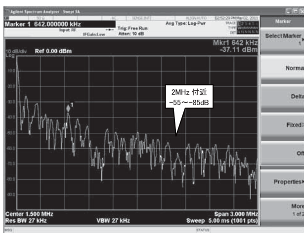
図 11 アイドリング時の FPGA のイズ(上)と演算時の FPGA のノイズ(下)の比較
