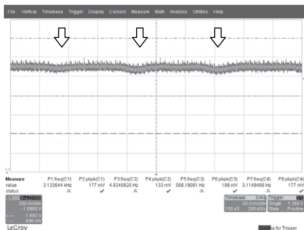
図8 直径5mmの気泡による透過受信電圧の変化
