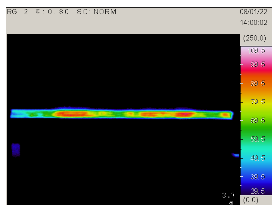
図2 熱画像，起電点を中央にとった場合
