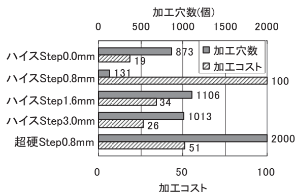
図 3 SUS304 加工時の工具寿命と加工コスト
