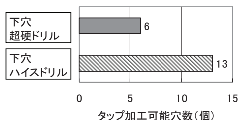
図 10 下穴加工とタップ加工可能穴数
