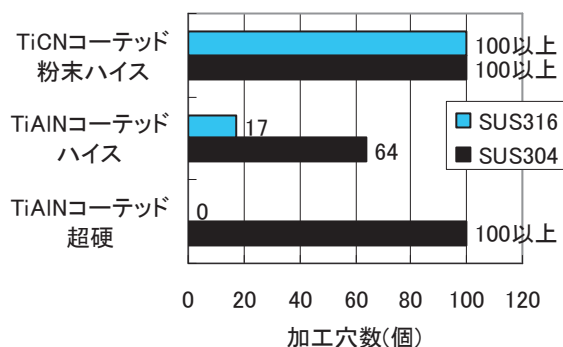
図 4 SUS304 と SUS316 の工具寿命
