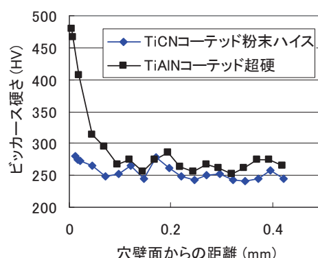
図 9 下穴の加工硬化
