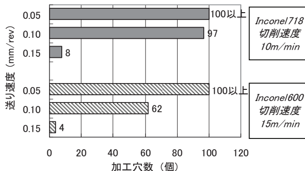
図 5 Inconel718 と Inconel600 の工具寿命
