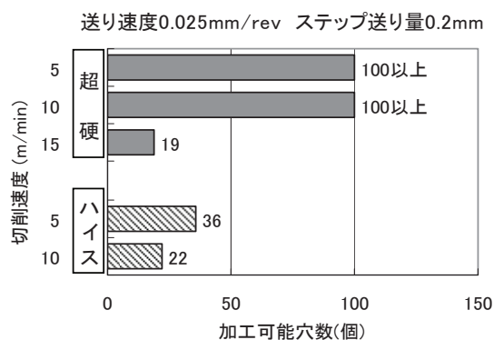
図 7 Inconel625 の工具寿命
