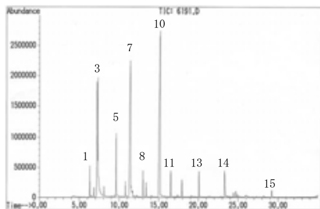
図1 正常な塩漬シロウリ臭い成分のトータルイオンクロマトグラム
