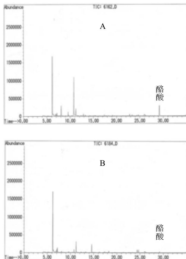
図 4 水さらし及びアルカリ浸漬後の塩漬シロウリ臭い成分のトータルイオンクロマトグラム
