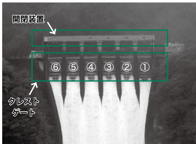
開閉装置全景
