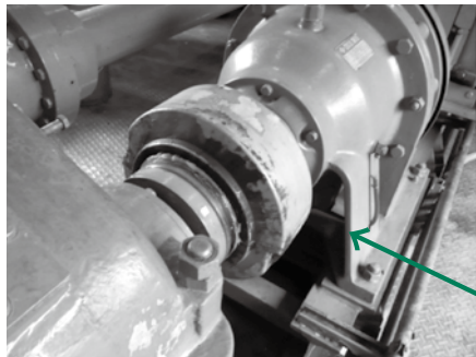
カップリング部の塗装劣化
