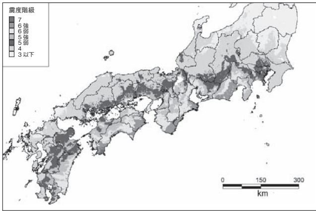
南海トラフの西側が震源地となった場合の震度分布図
