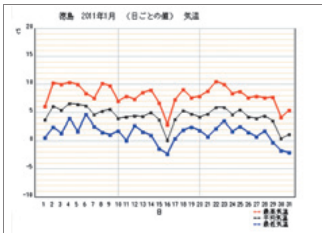
図1 徳島観測所の1月の気温
