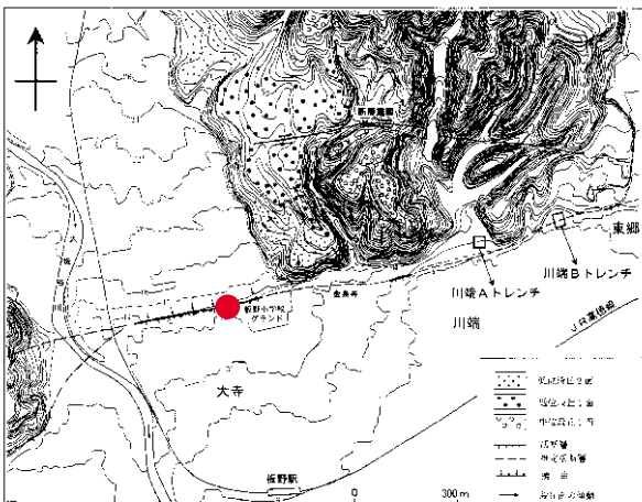
図1 板野町周辺の断層変位地形(森野ほか、2001)
